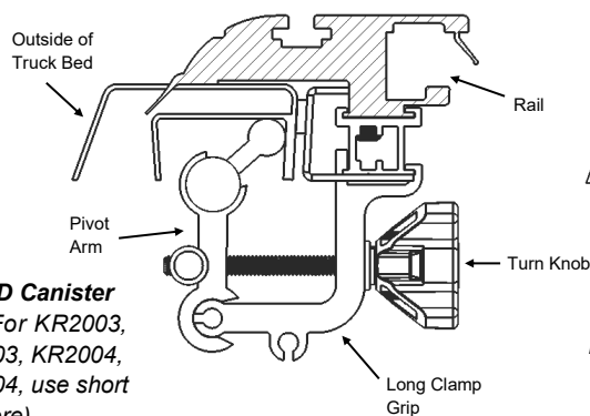
FIG. 7E Tailgate End
